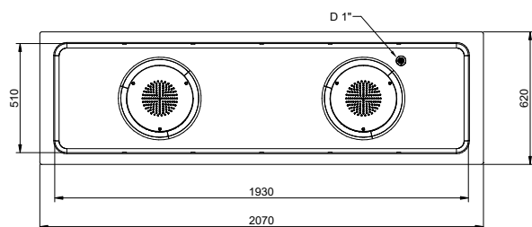
Topp
